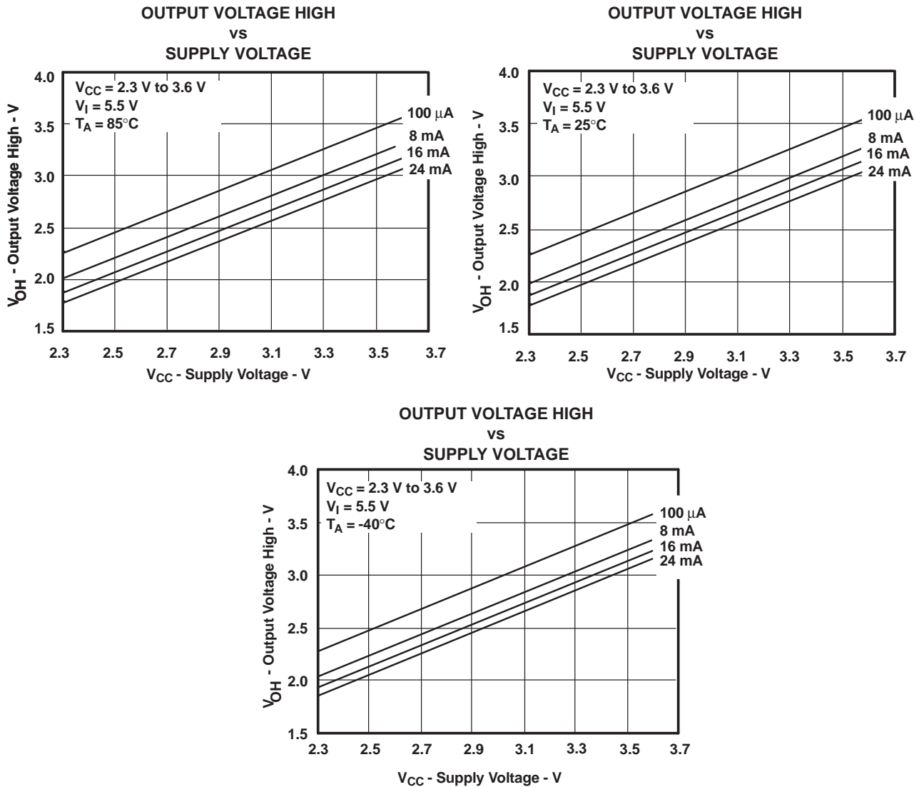
Figure 4. V_{OH} Values
