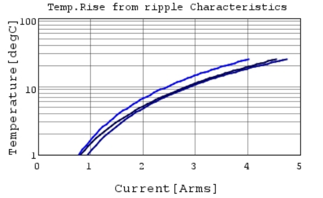
■ KRM55TR72A106MH01 Temp.rise — 50kHz
