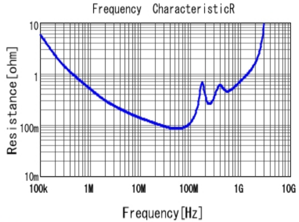
■ GA355DR7GF472KW01 R DCOV, 25degC
